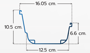
ขนาดหน้าตัดรางน้ำฝนไวโวนิล
